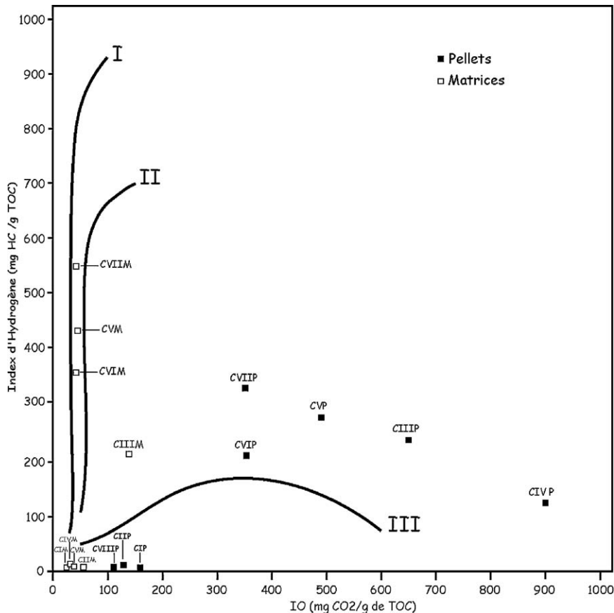
Fig. 2. Diagramme IH-IO montrant la position des points représentatifs de la MO des pellets et des matrices des sédiments phosphatés de la série de Ras-Draâ.
