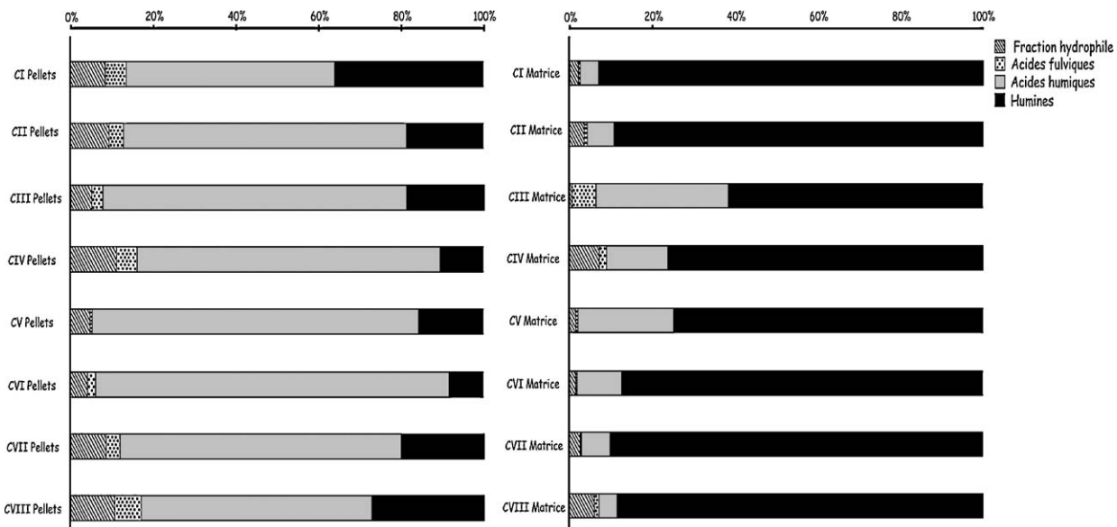
Fig. 3. Teneur en CO, en % du COT dans la somme des quatre fractions séparées HY + AF + AH + HU (COTfr).
