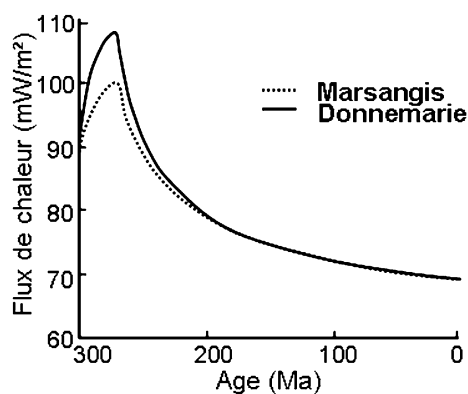
Fig. 2. Courbe d'évolution du flux de chaleur surfacique pour deux puits du bassin de Paris.
