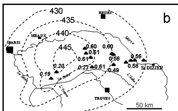
0.61 : Rapports d'isomérisation S/R des C 31 hopanes 0.19 : taux de transformation pour le Toarcien inférieur --- Courbes d'iso T max déterminées par [8] pour le Toarcien inférieur
