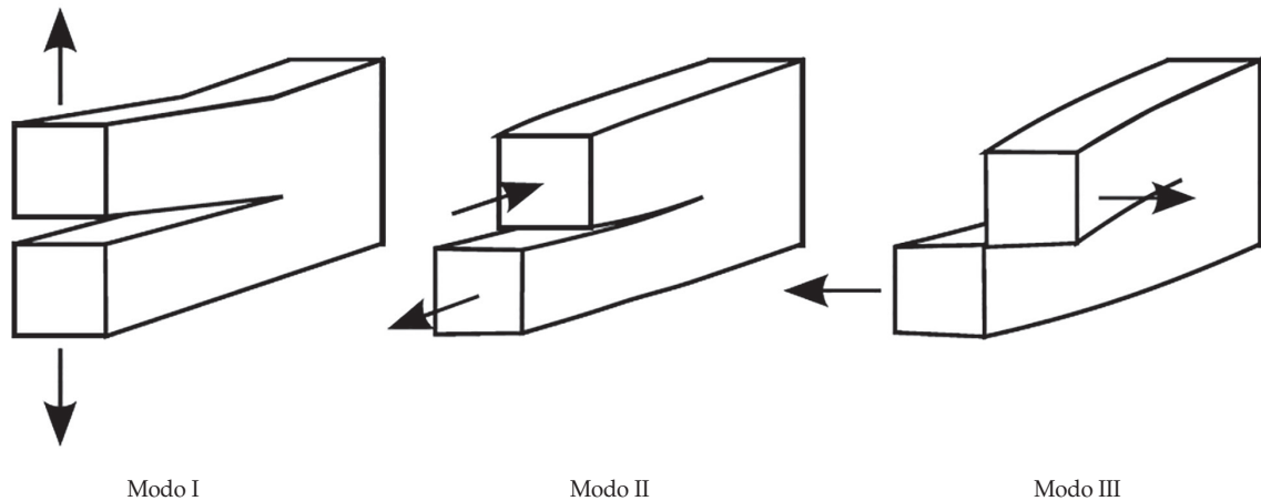
Figura 2 – Modos básicos de carregamento de um sólido fendido.
