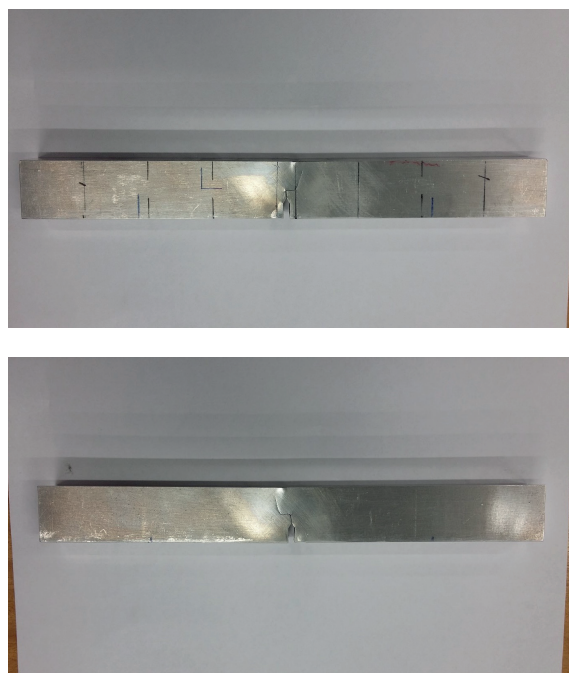
Figura 5 – Exemplo de desvio da direcção de propagação de uma fenda devido a alteração da razão modo I / modo II: provete de flexão em 4 pontos de AA 6082 T6 ensaiado na FEUP por J. Baganha Marques, 2017.
