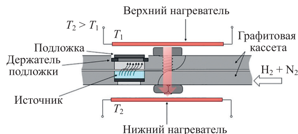
Рис. 1. Схематическое изображение процесса массопереноса в методе близкого переноса через тонкую газовую зону в поле температурного градиента: где T_1 и T_2 — температура верхнего и нижнего нагревателя Fig. 1. Schematic representation of the mass transfer process in the method of close transfer through a thin gas zone in the temperature gradient field: where T_1 and T_2 are the temperatures of the upper and lower heaters
