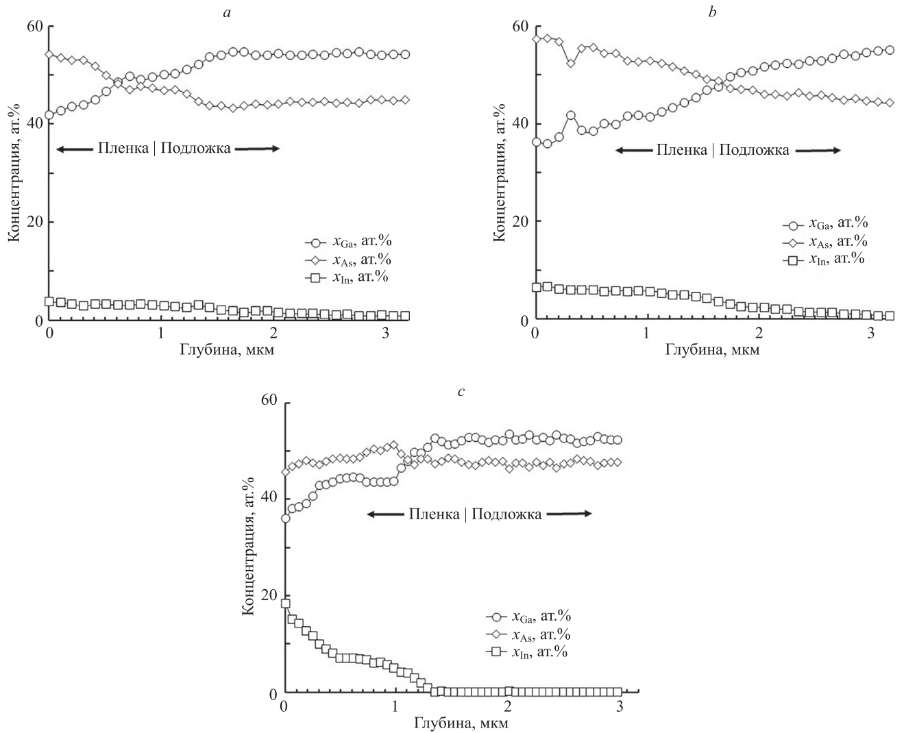
Рис. 3. Профиль концентрации по глубине вдоль скола пленок \text{Ga}_{1-x}\text{In}_x\text{As} , выращенных при T = 1123 \text{ K} и G = 30 \text{ K/cm} для концентраций индия x_{\text{In}} : 10 % (a), 20 % (b) и 30 % (c)
