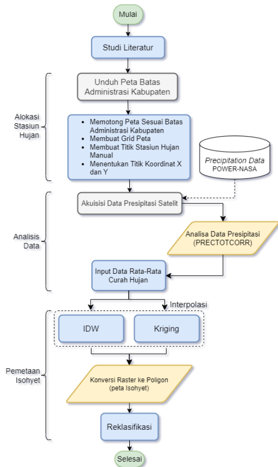
Gambar 1. Kerangka Penelitian
