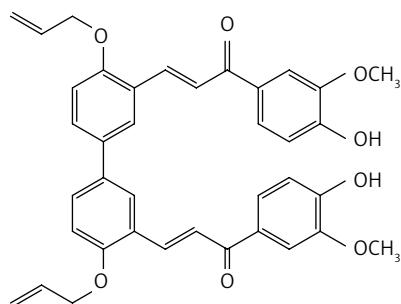
Figure 16. (E)-3-(4,4'-bis(allyloxy)-3'-((E)-3-(3-hydroxy-4-methoxyphenyl)-3-oxoprop-1-en-1-yl)-[1,1'-biphenyl]-3-yl)-1-(4-hydroxy-3-methoxyphenyl)prop-2-en-1-one (29)
