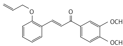
Figure 17. (E)-3-(2-(allyloxy)phenyl)-1-(3,4-dimethoxyphenyl)prop-2-en-1-one (30)
