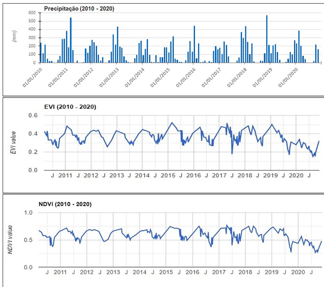
Figura 2. Variabilidade dos IVs (EVI e NDVI) em relação aos regimes de precipitação (2010 – 2020) / Variabilidad de los IV (EVI y NDVI) en relación con los regímenes de lluvia (2010 - 2020)
