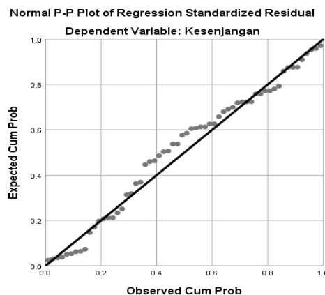
Gambar 3. Grafik P-Plot Uji Normalitas
