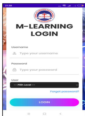
Gambar 2. Tampilan Login
