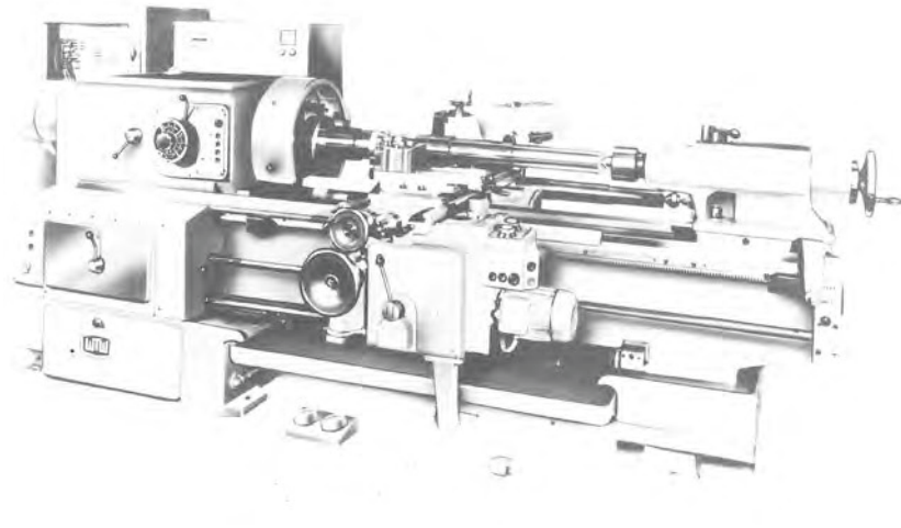
Automatisierte DZ 500/IV mit Steckerfeldsteuerung (1962)
