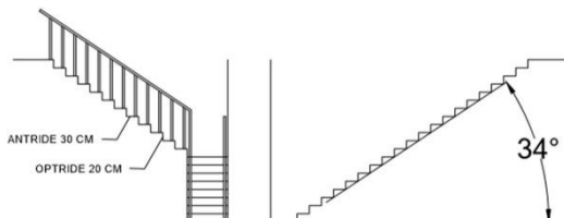
Gambar 4.10. Exsisting tangga di dalam masjid At-taqwa
