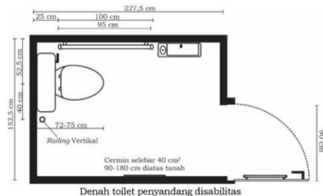
Gambar 4.22. ruang dalam toilet penyandang disabilitas yang dilengkapi dengan pegangan rambat Sumber : Permen PU dan Perumahan Rakyat nomor 14/ PRT/M/2017
