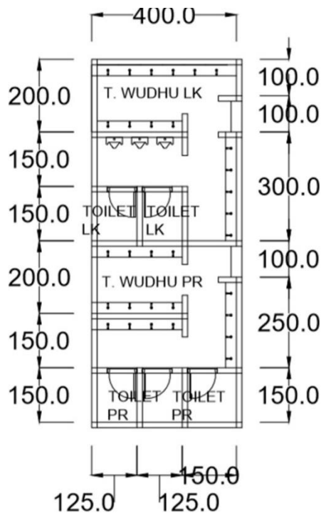
Gambar 4.13. existing tempat wudhu masjid At-taqwa
