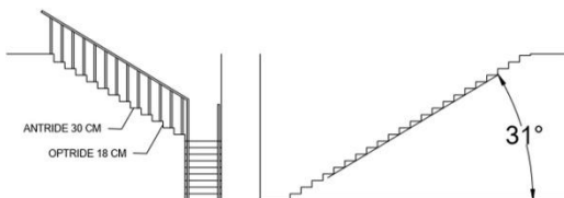
Gambar 4.18. rencana tangga di dalam masjid
