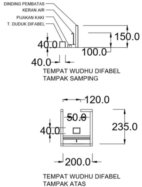
Gambar 4.24. rencana toilet masjid At-taqwa
