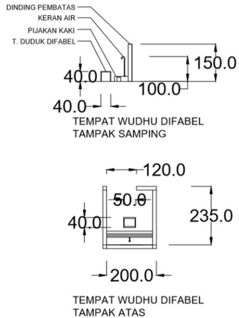
Gambar 4.21. rencana tempat wudhu difabel pada masjid At-taqwa
