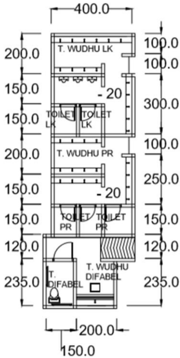
Gambar 4.20. rencana tempat wudhu masjid At-taqwa
