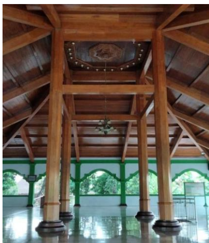
Gambar 3 4 pilar kayu jati pada Masjid Jami' Sunan Abinawa pada bagian luar
