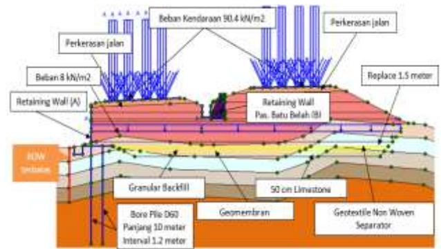
Gambar 3. Pemodelan Plaxis
