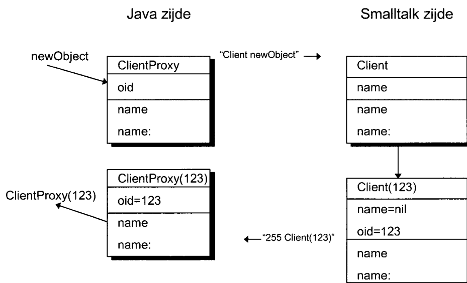
Figuur 16 Klasse methode conversie
