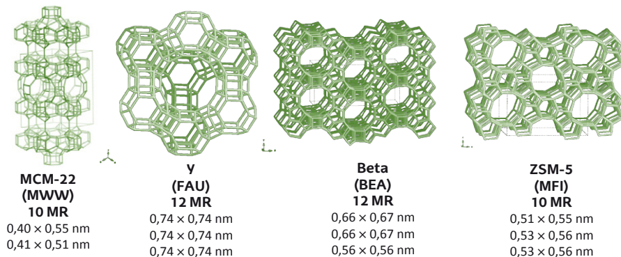
7. irudia. Etilenoaren oligomerizaziorako erabilitako ohiko zeotipoak [32].
