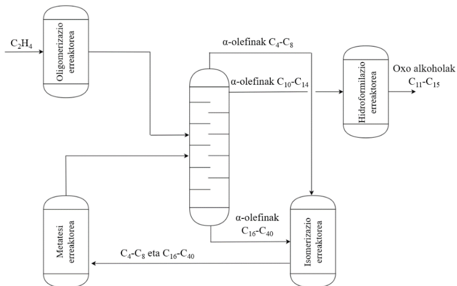
4. irudia. SHOP prozesuaren diagrama [23].
