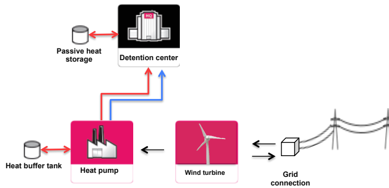
Figuur 1 Smart micro grid scenario met een windturbine en een warmtepomp, welke flexibel is door gebruik van warmte opslag
