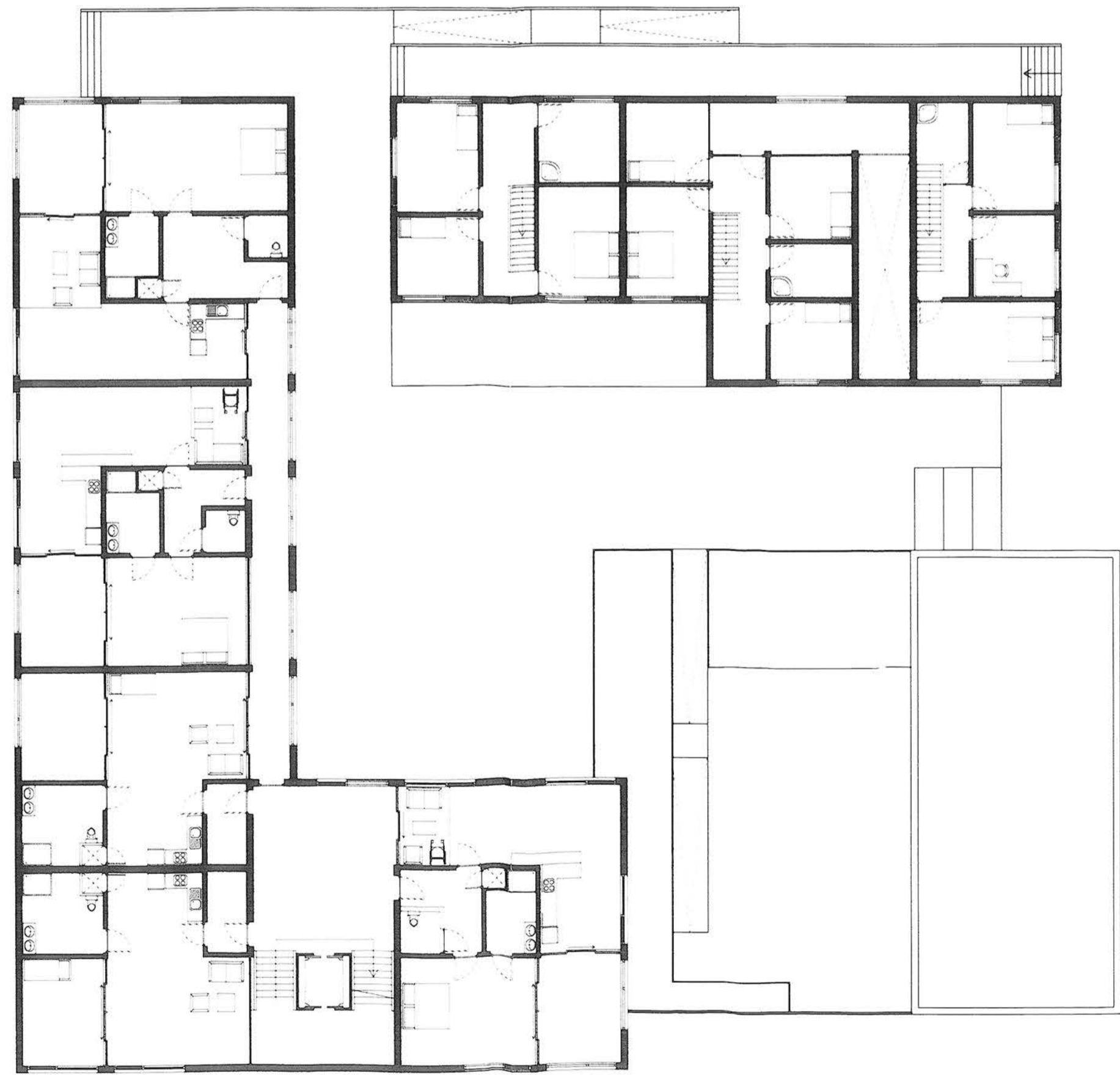
Vloer 3, schaal 1:200
