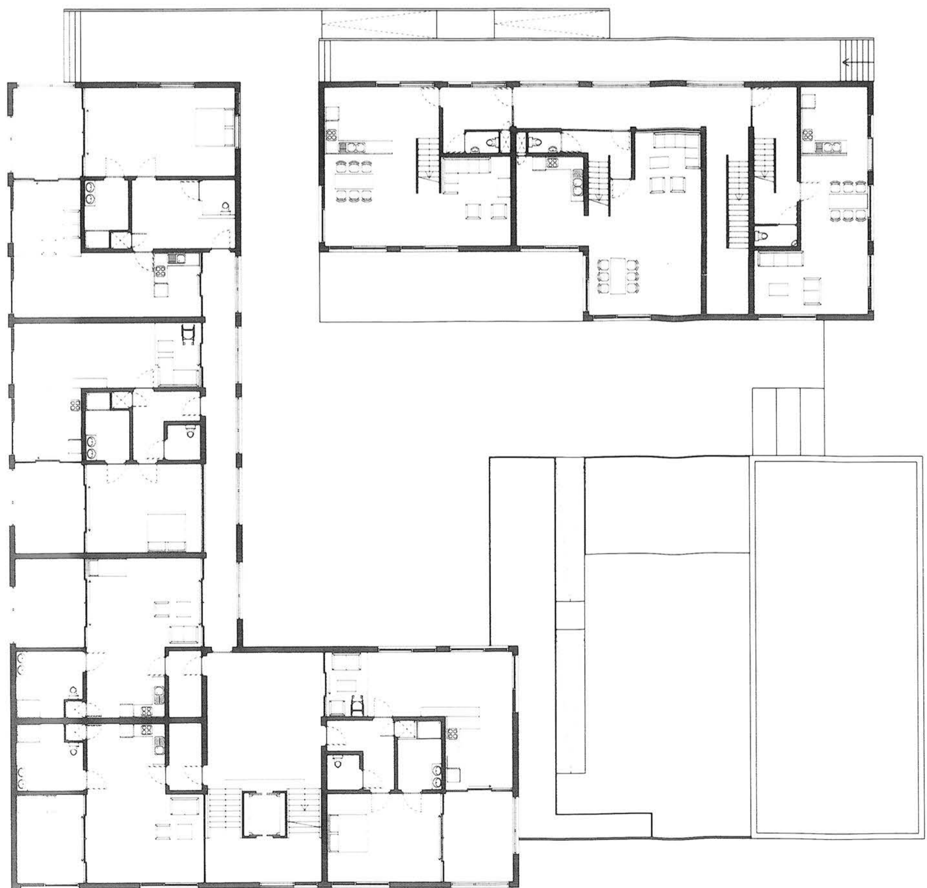
Vloer 2, schaal 1:200
