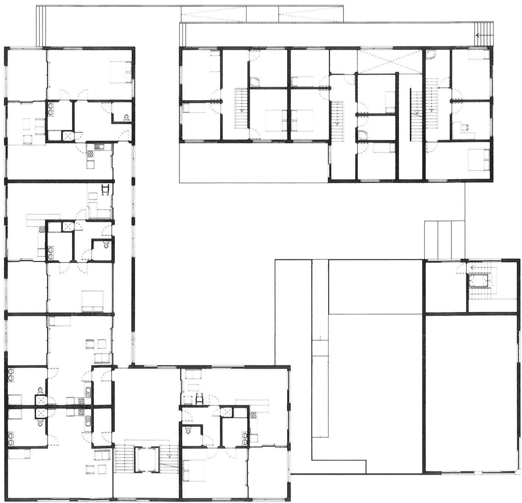
Vloer 1, schaal 1:200
