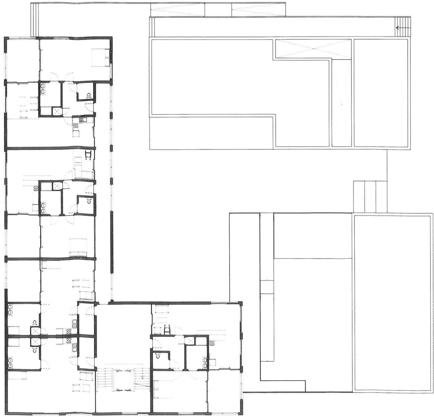
Vloer 4, schaal 1:200
