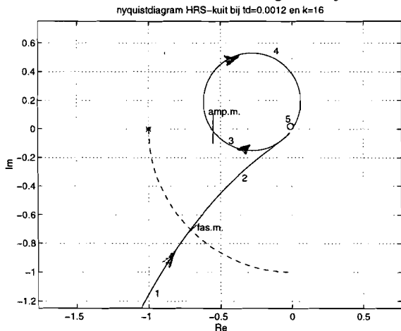
Figuur B8.3 Kuitspijermeting
