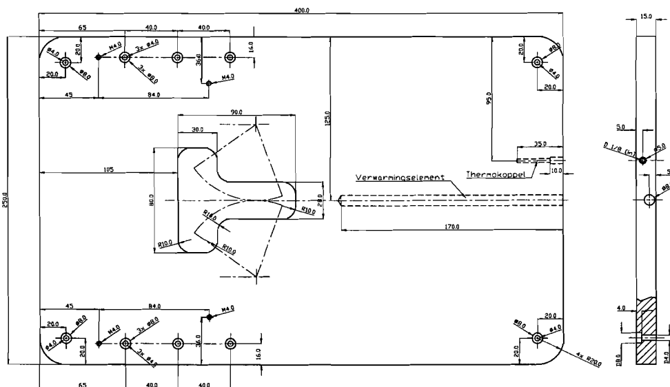
Figuur B12.2 De dimensies van het meetplateau van de staartfixatie voor de rat (prototype 1), schaal 1:4
