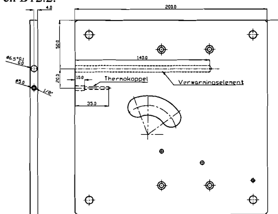
Figuur B12.1 De dimensies van het meetplateau van de staartfixatie voor de muis (prototype 2), schaal 1:4
