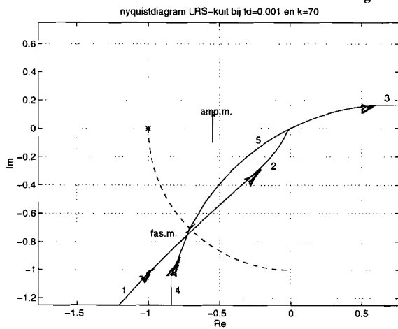
Figuur B8.5 Kuitspijermeting
