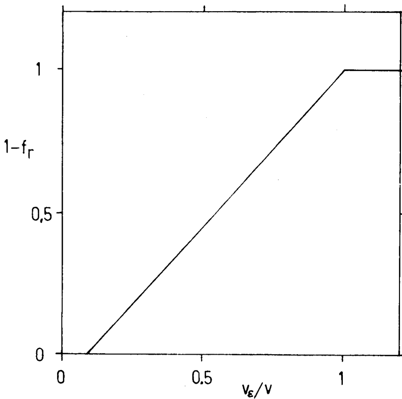
Fig. 4. De fraktie van de doorgelaten bundel als funktie van de inverse gereduceerde grootheid v_\epsilon/v . Voor snelheden groter dan v_\epsilon vindt afkapping plaats.
