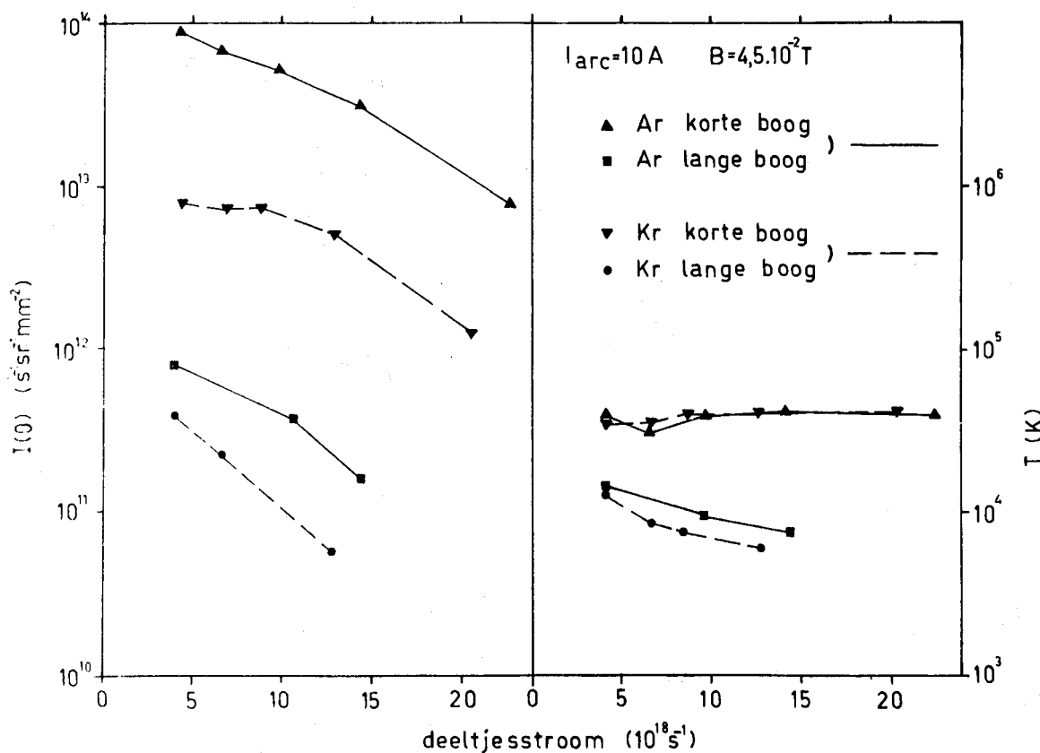
Fig.48. Een overzicht van de resultaten van de metingen aan Ar en Kr voor beide boogconfiguraties.
