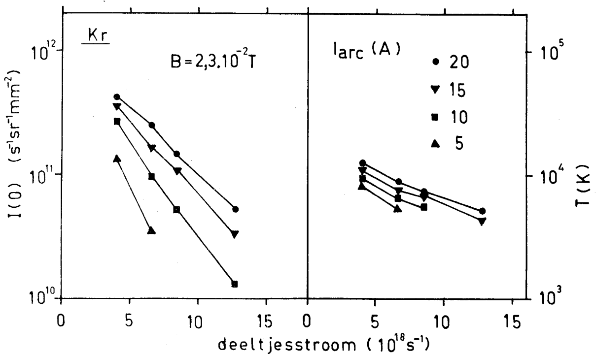
Fig. 57. Als in figuur 56 maar nu met een magnetische inductie van 2,3 \cdot 10^{-2} \text{ T} .
