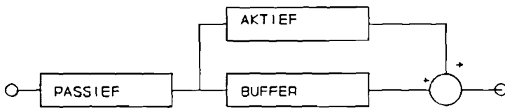
Fig. 2.4 Blokschema van de integrator
