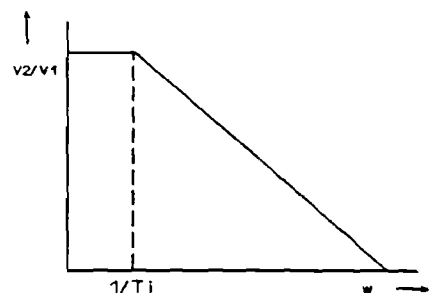
Fig. 2.6 Bodediagram van de integrator
