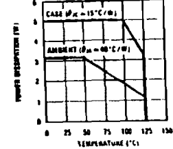
LH0063 Power Dissipation
