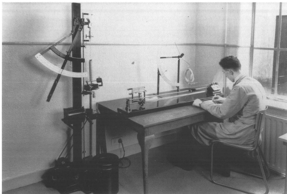
Afb. 14. De Nedcos had een eigen laboratorium, waarover geen nadere bijzonderheden bekend zijn. Hier een laborant bij het nemen van trekproeven voor het bepalen van de garenssterkte, hoogstwaarschijnlijk in 1950.
