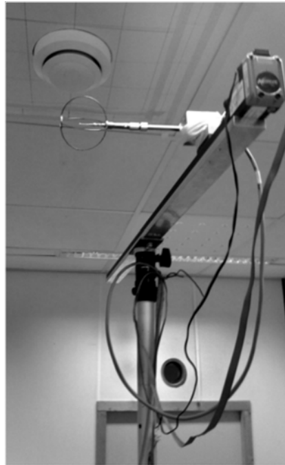
-Figuur 1- Meetopstelling voor het meten van het snelheidsprofiel van een van de onderzochte toevoerventielen (axiaal)
