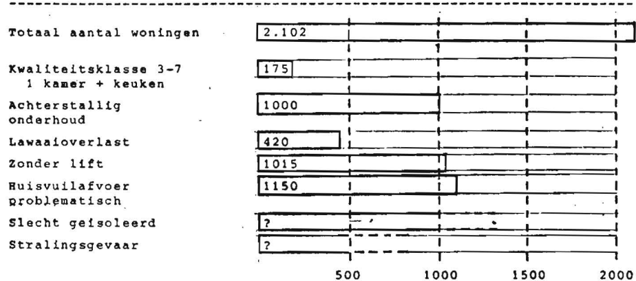
SCHEMA 3:1
