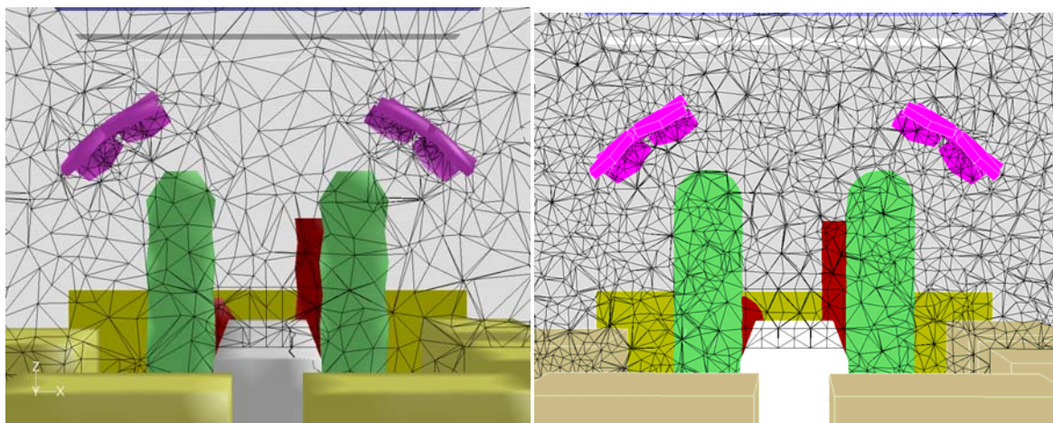
Figuur 2. Voorbeelden van verschillende celgroottes (links: 0.20 m; rechts: 0.10 m).
