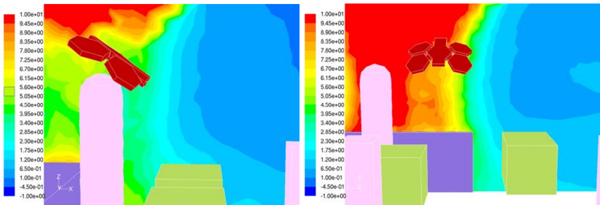
Figuur 7. Voorbeeld van een berekende protectiefactor voor een verticale doorsnede in de operatiekamer (links: instrumenttafel aan de linkerzijde van de operatietafel; rechts: instrumenttafel aan het voeteneinde van de operatietafel).
