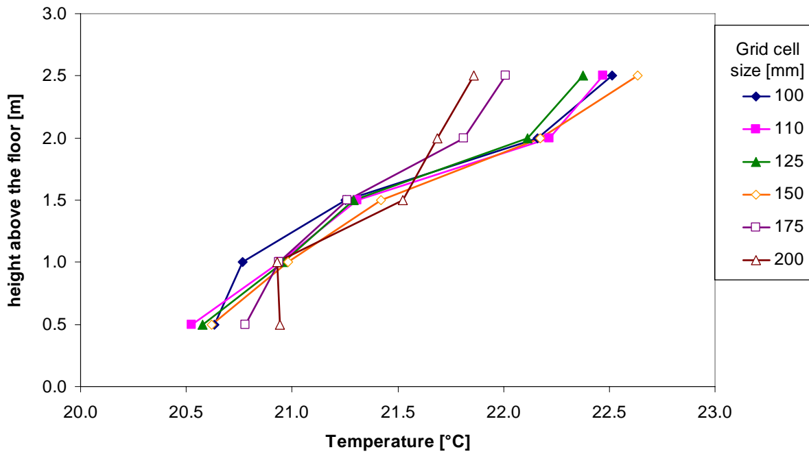
Figuur 3. Verticale temperatuur gradiënt in de periferie van de kamer voor verschillende celgroottes.
