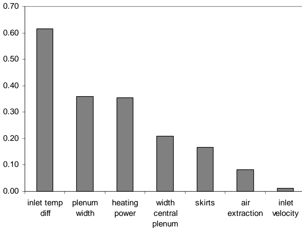
Figuur 5. Absolute waarde van de correlatiecoëfficiënt tussen de protectiefactor op de operatietafel en 7 verschillende ontwerpparameters.
