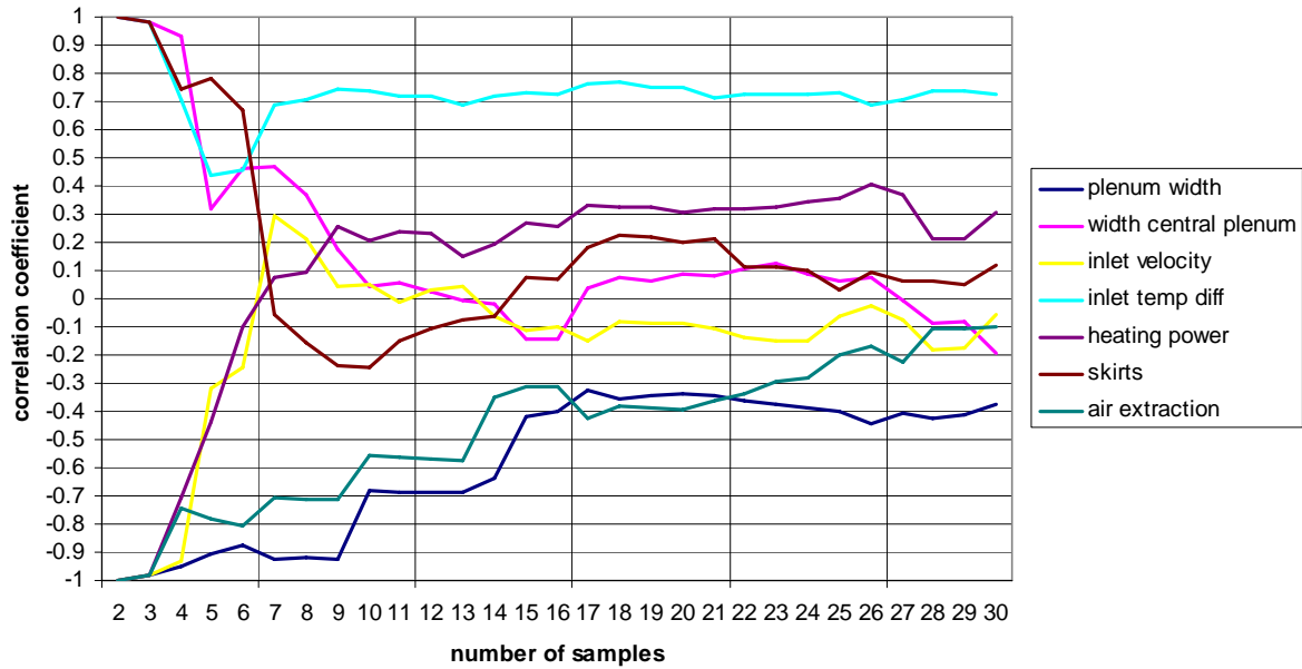
Figuur 6. Ontwikkeling van de correlatiecoëfficiënt van de verschillende parameters in de Monte Carlo analyse.
