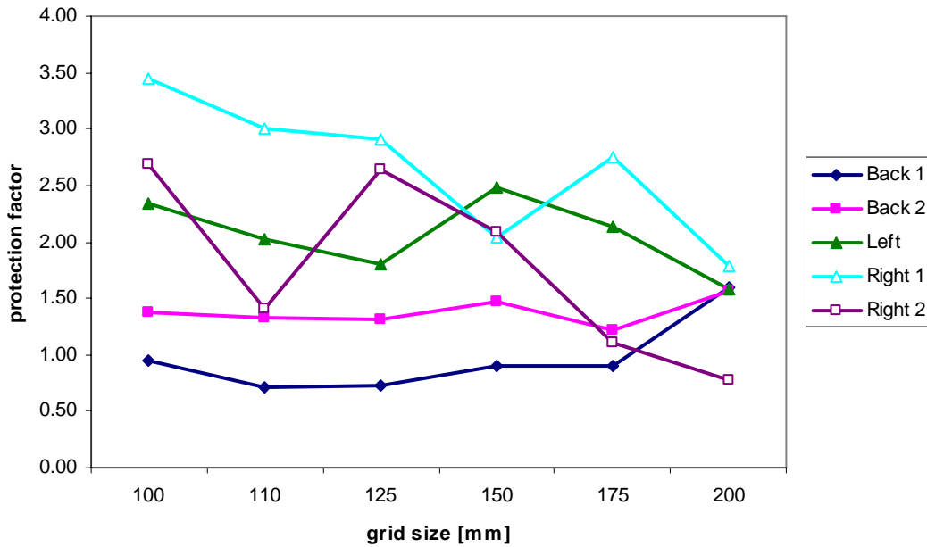
Figuur 4. Protectiefactor op de instrumenttafels als functie van de celgrootte.
