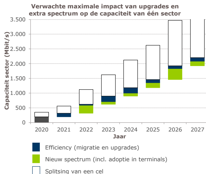
Figuur 16 Impact van upgrades op capaciteit in mobiele netwerken (bron: modellering Dialogic; zie Bijlage 1) 28
