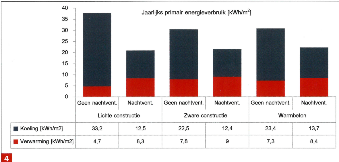
4 Het jaarlijks primaire energieverbruik [kWh/m²] voor de drie constructietypes met en zonder nachtventilatie
