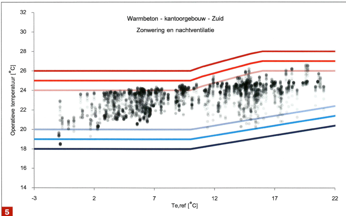
5 De operationele temperatuur [°C] als functie van de referentietemperatuur [°C]. De grafiek toont de uren wanneer personen aanwezig waren in het kantoorgebouw
