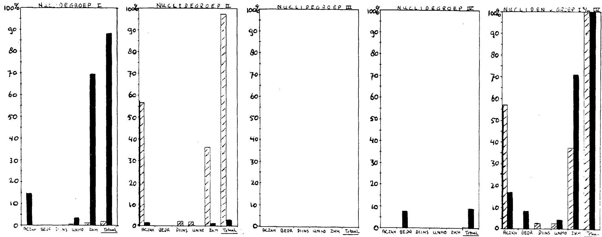
FIGUUR 3.6. Relatieve verdeling van de toegepaste hoeveelheden radioactieve stoffen in de vorm van open bronnen per nuclidegroep (per gebruikerscategorie) Zwarte staven hebben betrekking op activiteit uitgedrukt in curie. 100% komt overeen met ongeveer 2000 curie. Gearceerde staven hebben betrekking op toxiciteit uitgedrukt in ALI-eenheden. 100% komt overeen met ongeveer 1,6 \cdot 10^6 ALI-eenheden. Bijdragen kleiner dan 0,5% zijn niet weergegeven.
