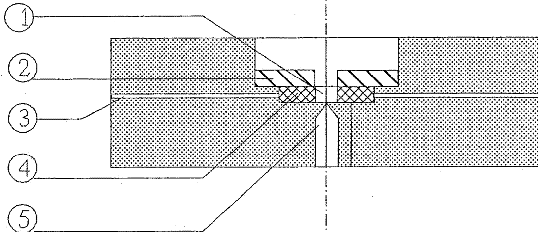
Figuur 5.2: Doorsnede meetblok 1:proefstukje, 2:perspex deksel, 3:leiding spoelvoeistof, 4:glasfilter, 5:naaldhouder
