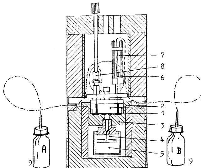
Figuur B2.1: Knauer osmometer
