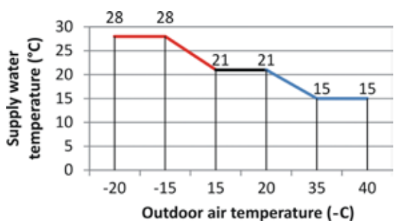
-Figuur 4- Watertoevoertemperatuur als functie van de buitentemperatuur
