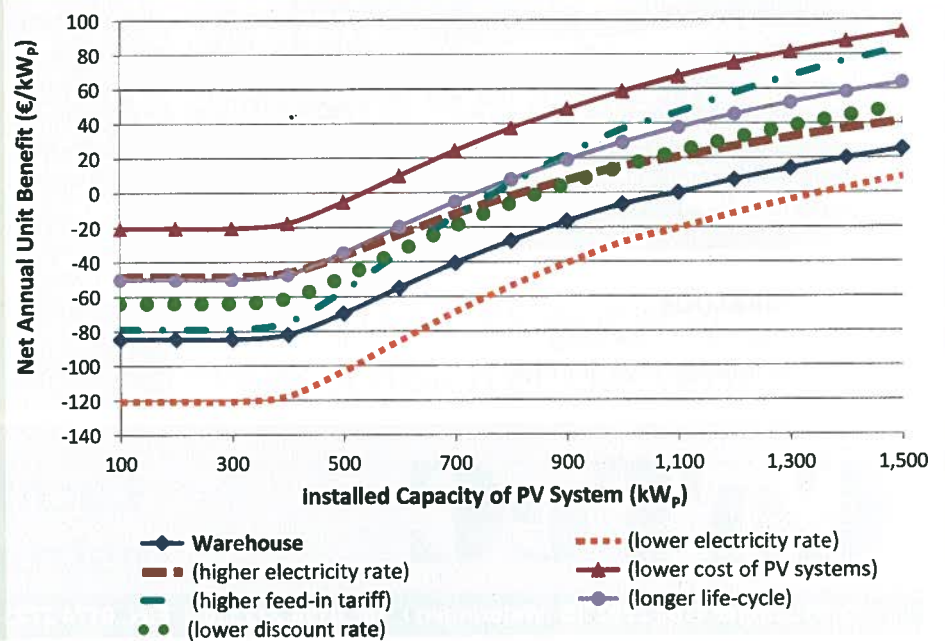
-Figuur 2- Jaarlijkse opbrengst (per kW p ) van pv-systemen bij variaties in economische parameters voor een opslagloods in Palermo met de netto TLV-regeling
