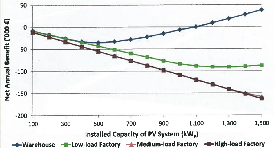
-Figuur 1- Jaarlijkse winst bij de netto TLV-regeling
