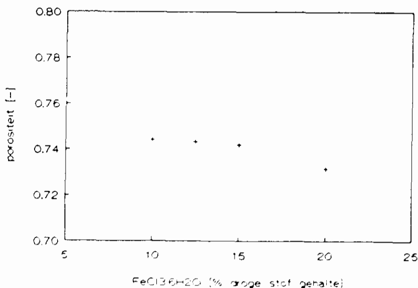
Figuur 7. Porositeit tegen de concentratie \text{FeCl}_3 \cdot 6\text{H}_2\text{O} (200 ml slib, 20% \text{Ca}(\text{OH})_2 , P = 766,64 \text{ Pa} )
