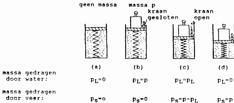
Figuur 2. Schematische weergave van het Terzaghi-model
