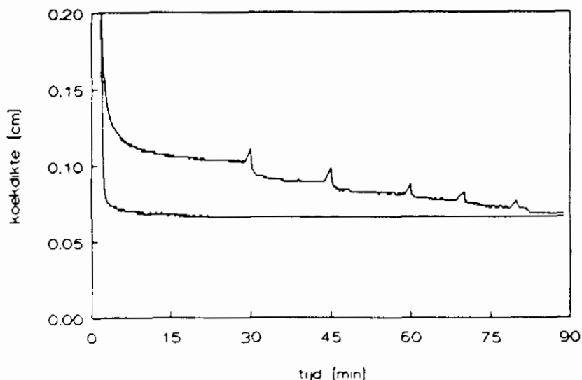
Figuur 6. Koekdikte tegen de tijd bij opleggen druk in één meerstapsfunctie
