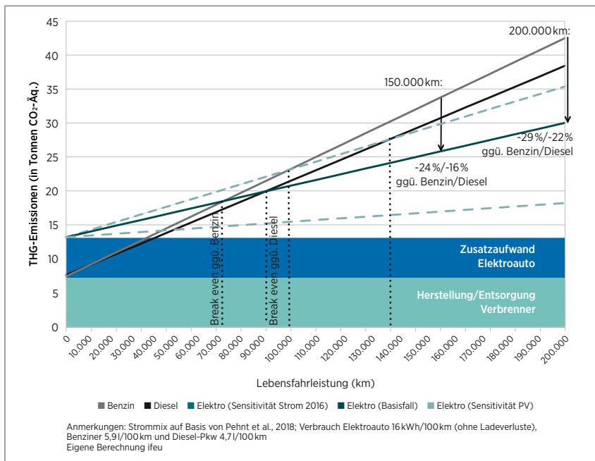
Abbildung 41: Treibhausgasemissionen von Benzin, Diesel und Elektroautos in Abhängigkeit der CO 2 -Emissionen aus der Stromerzeugung und der Lebensfahrleistung Quelle: Agora Verkehrswende 2019
