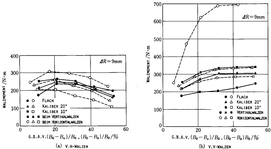
Bild. 17 Zusammenhang zwischen dem Gesamtbreitenabnahmenverhältnis und dem Vertikal- und Horizontalwalzmoment (a) beim V. H-Walzen und (b) beim V.V-Walzen
