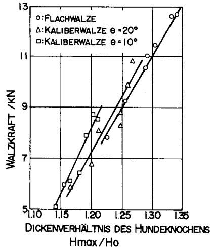
Bild. 5 Zusammenhang zwischen dem Hundeknochendickenverhältnis und der Walzkraft
