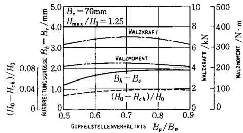
Bild. 10 Rechnerisches Ergebnis über den Zusammenhang zwischen dem Gipfelstellenverhältnis und den Walzeigenschaften beim Horizontalwalzen
