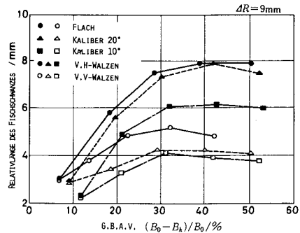
Bild. 16 Vergleich zwischen dem V.H-Walzen und V.V-Walzen über die Relativlänge des Fischschwanzes
