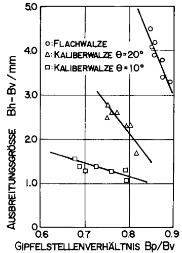
Bild. 7 Zusammenhang zwischen dem Gipfelstellenverhältnis und der Ausbreitungsgröße
