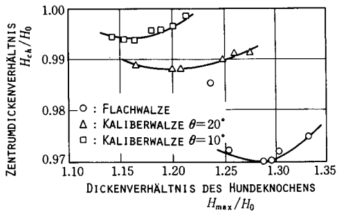
Bild. 6 Zusammenhang zwischen dem Hundeknochendickenverhältnis und dem Zentrumsdickenverhältnis
