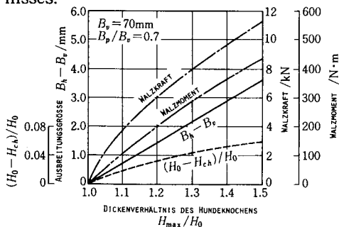
Bild. 9 Rechnerisches Ergebnis über den Zusammenhang zwischen dem Hundeknochendickenverhältnis und den Walzeigenschaften beim Horizontalwalzen
