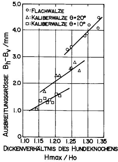
Bild. 4 Zusammenhang zwischen dem Hundeknochendickenverhältnis und der Ausbreitungsgröße
