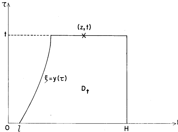
Fig. 3. Domain D_t .
