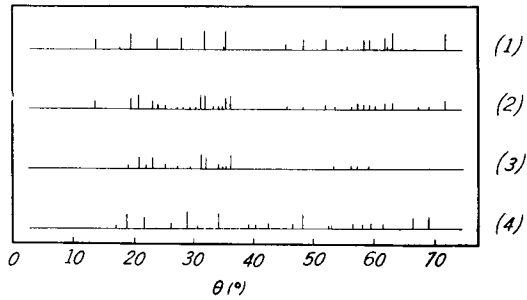
(1) Ni 3 S 2 (2) Ni 6 S 5 (3) Ni 7 S 6 (4) NiS
