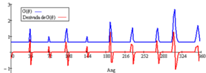
Figura 7: Representación gráfica de la función G(\theta_i) y su derivada
