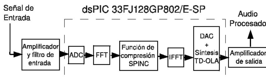
Figura 6. Esquema del dispositivo propuesto.
