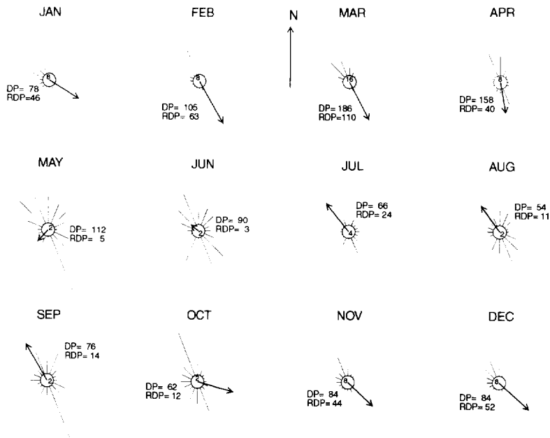
Fig. 21. Monthly sand roses for Akron, Colorado.
