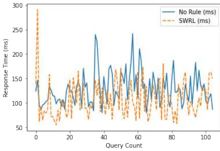
Fig. 20. Evaluation 3 visualisation
