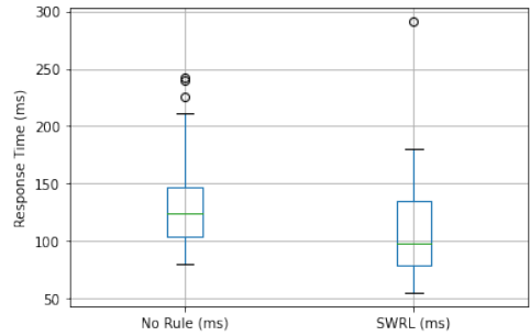
Fig. 21. Evaluation 3 boxplot
