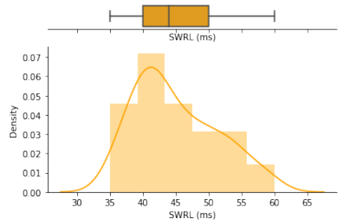
Fig. 16. Evaluation 2 boxplot
