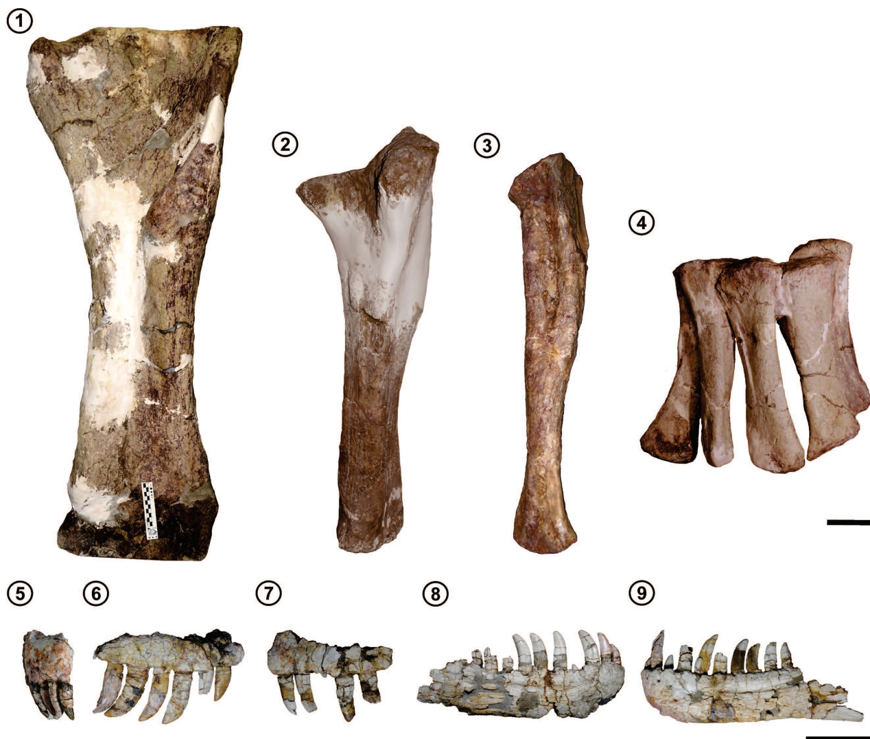
Figura 3. Algunos materiales holotípicos de dinosaurios del MLP. 1–4, Argryrosaurus superbus (MLP 77-V-29-1). 1, húmero izquierdo en vista anterior; 2, ulna izquierda en vista anterolateral; 3, radio izquierdo en vista posterior; 4, metacarpo izquierdo en vista anterior. 5–9, Genyodectes serus (MLP 26-29); 5, premaxila izquierda en vista lateral; 6, maxila derecha en vista lateral; 7, maxila izquierda en vista lateral; 8, dentario derecho en vista lateral; 9, dentario izquierdo en vista lateral. Escala= 10 cm.
