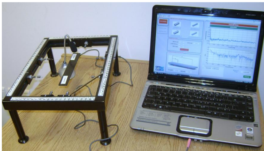
Figura 1: Soporte universal de cuerdas y sistema para medir la presión sonora.
