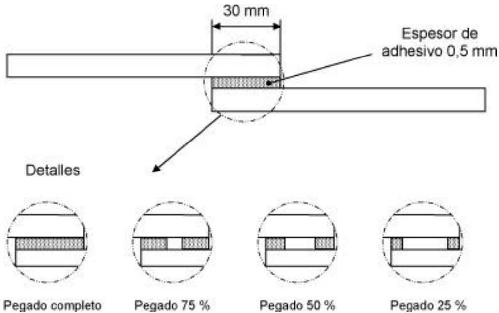
Figura 3 : Esquema de las vigas de aluminio EN AW 7075 total y parcialmente adheridas con epoxi.
