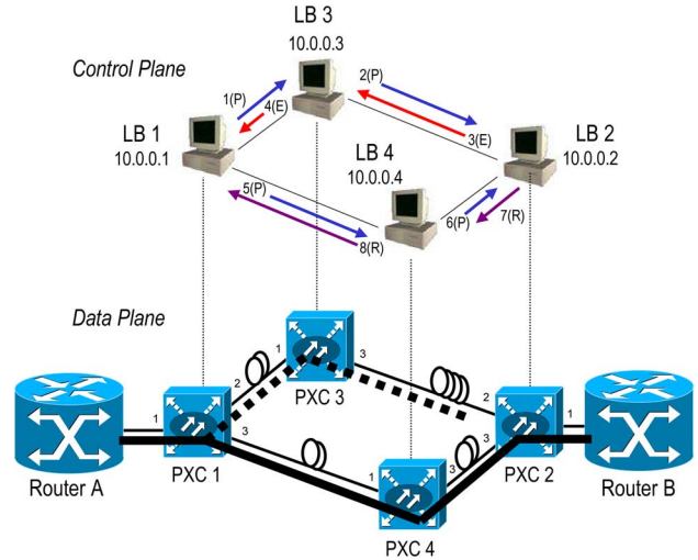
Fig. 17. Testbed implementing SA.
