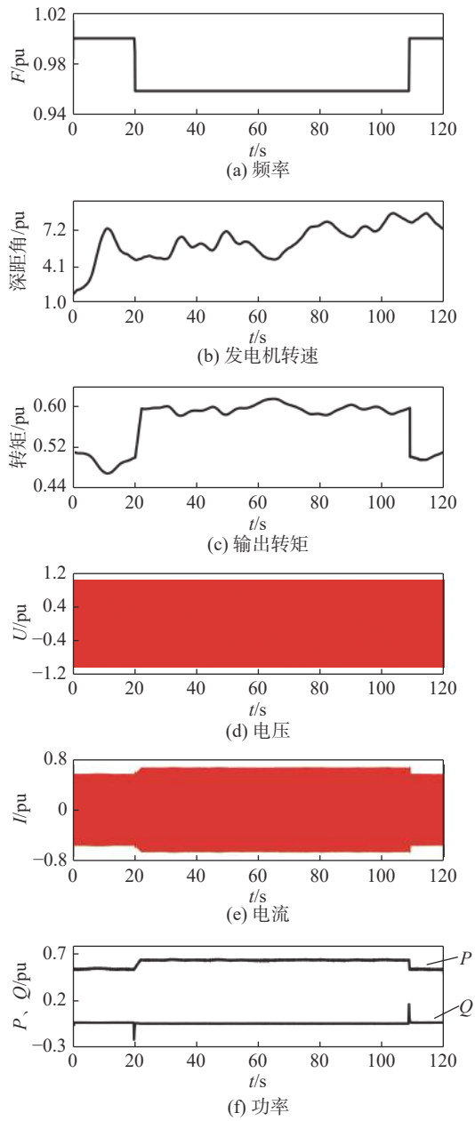
图 5 一次调频 50~48 Hz 波形图
