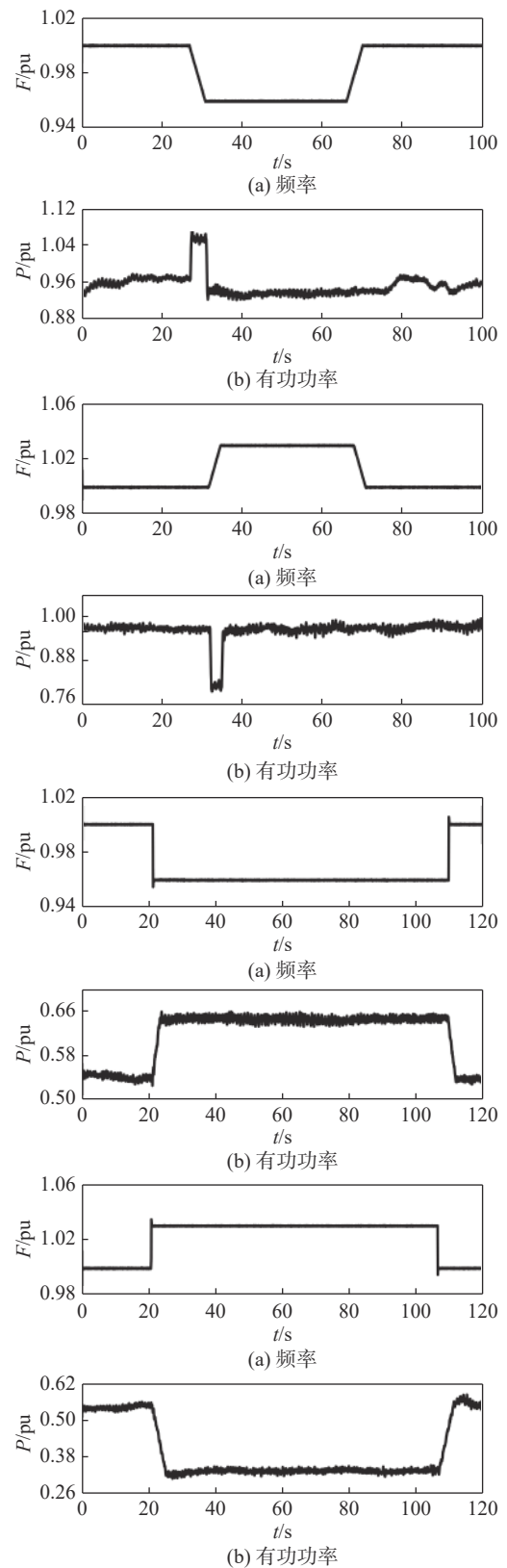
图 6 风电机组惯量响应及一次调频测试结果
