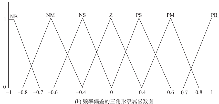
图 5 电压偏差和频率偏差的三角形隶属函数图
