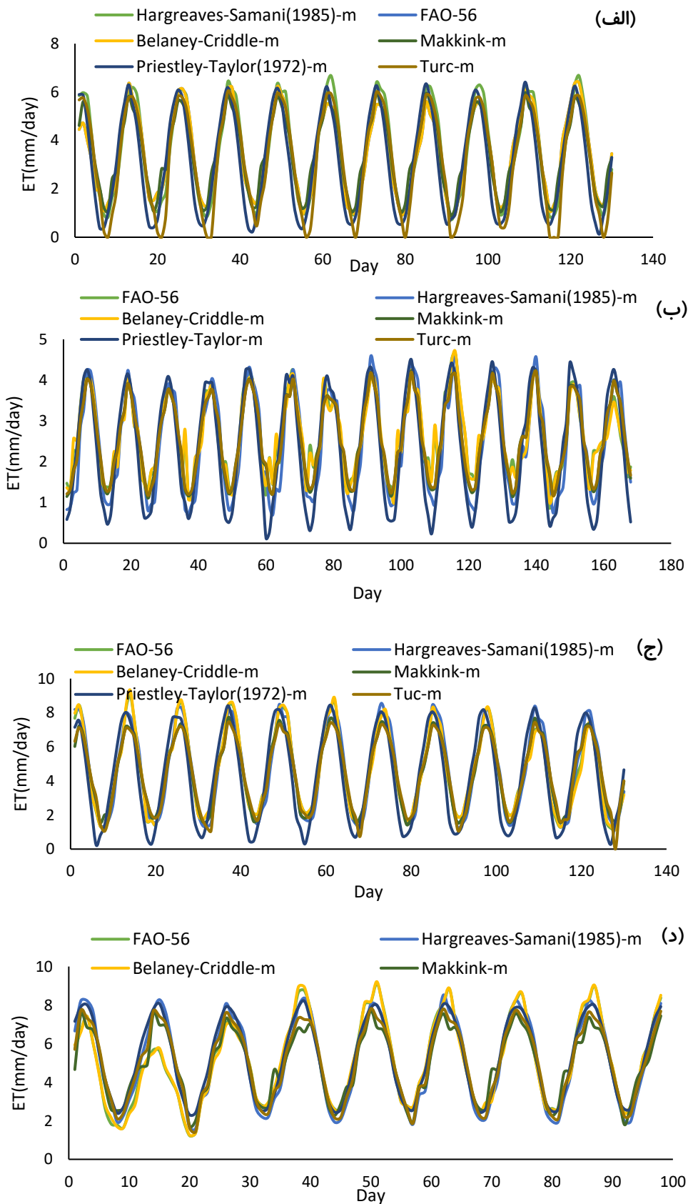
شکل ۲- روند برآورد تبخیر-تعرق روش‌های واسنجی شده نسبت به داده‌های مشاهداتی در ایستگاه‌های: الف) - ارومیه، ب) - رشت، ج) - مشهد، و د) یزد
