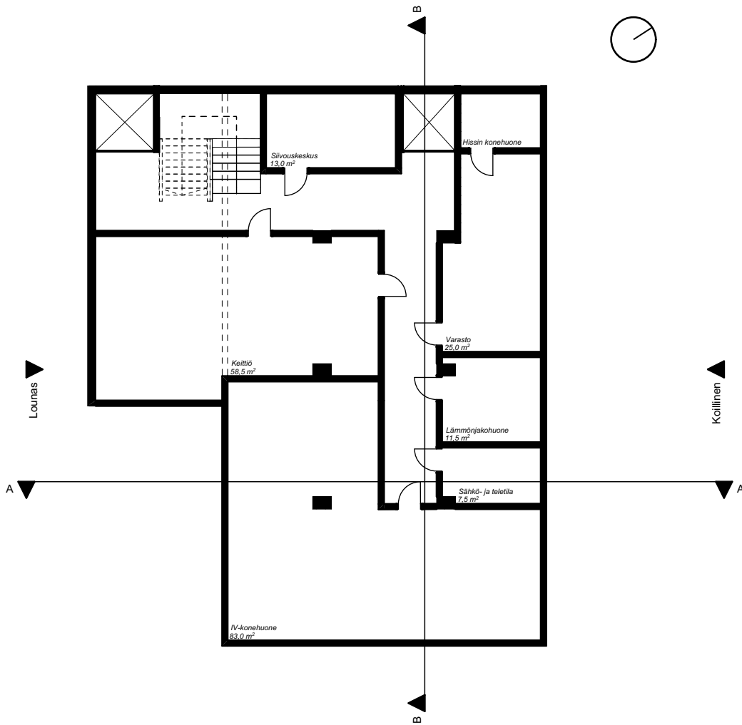
Kellarikerros 1:200
