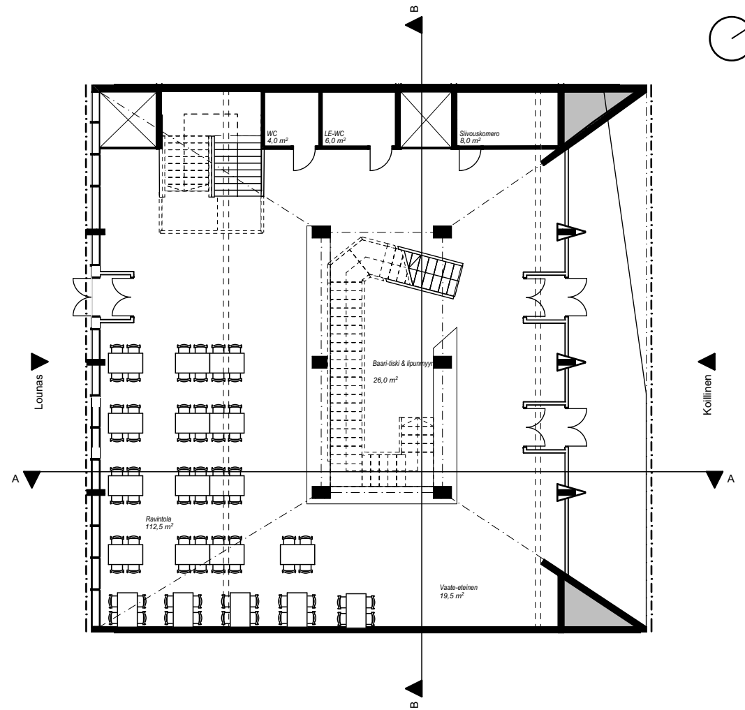
1. kerros 1:200
