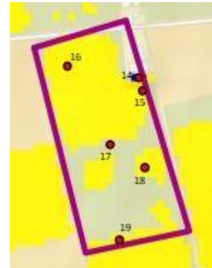
Figuur 7: SOC voorspelling op basis van Sentinel-2 beelden. Perceel 11, Dronten.
