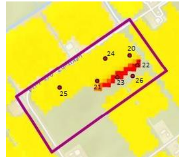
Figuur 9: SOC voorspelling op basis van Sentinel-2 beelden. Perceel 1, Biddinghuizen.
