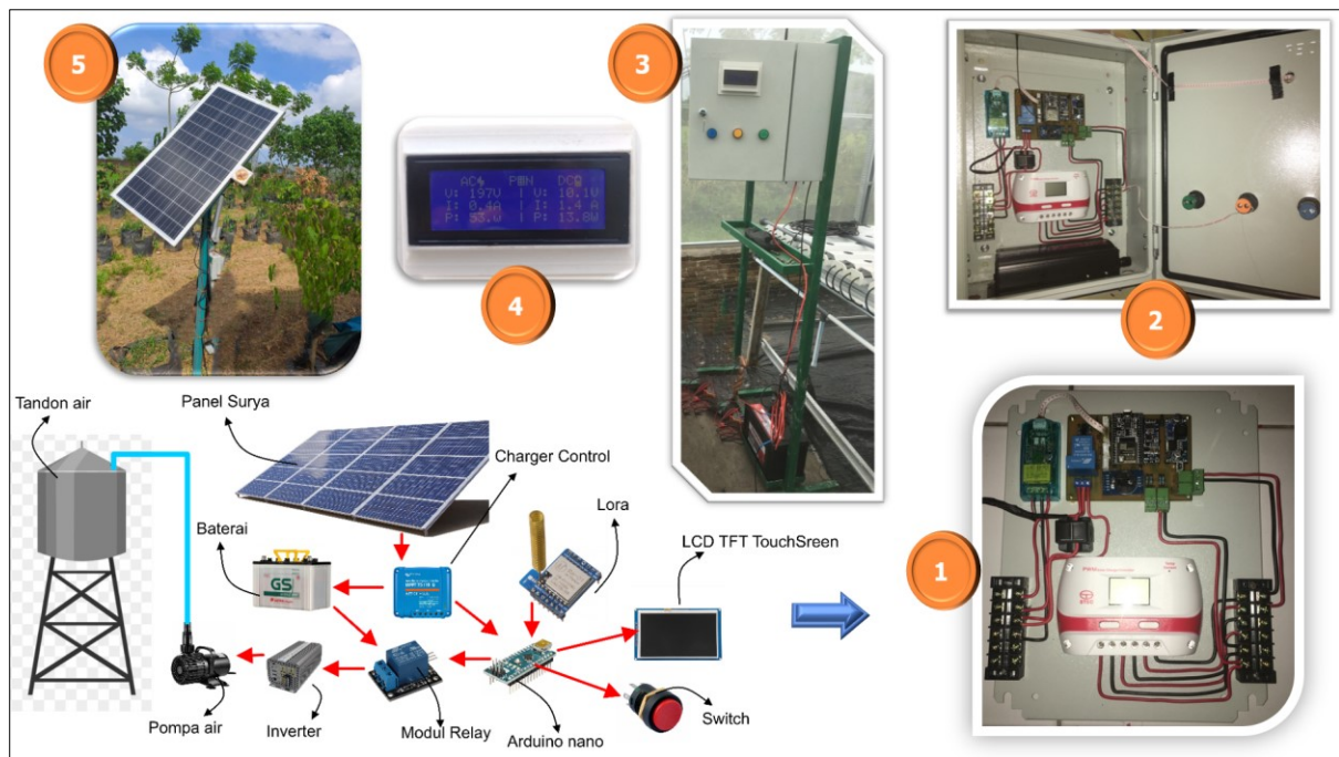
Gambar 1 Perangkat dan Tahapan Instalasi Sistem Pintar Kelistrikan SEIRS
