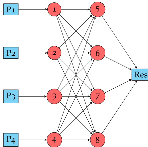
Figura 22: Modello di esecuzione DAG per il processo di Figura 3. I vertici azzurri sono i dati in input/output, mentre i vertici in rosso sono quelli che descrivono la computazione.
