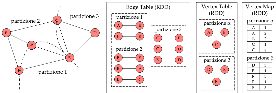
Figura 10: Esempio di vertex-cut con il grafo della Figura 5.
