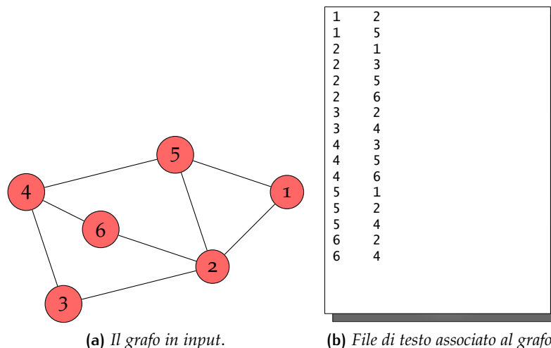
Figura 11: Il grafo semplice di Figura 5 con annesso il suo file descrittore. Per ogni arco del grafo ci sono due stringhe che lo rappresentano nelle due direzioni opposte.
