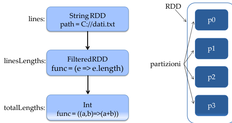
Figura 1: A sinistra, catena della lineage dei dataset RDD descritti nell'esempio. A fianco lo schema di un RDD con quattro partizioni.
