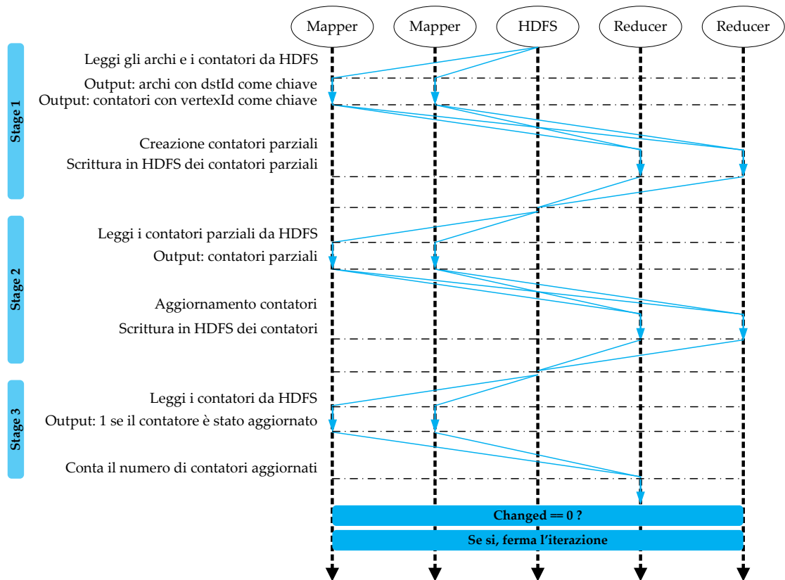
Figura 8: Schema del ciclo di operazione di HADI nella sua implementazione parallela.
