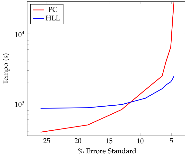
Figura 14: Confronto tra i tempi di esecuzione di HADI-Spark con HyperLogLog e con ProbabilisticCounter. Il grafo in ingresso è orkut .
