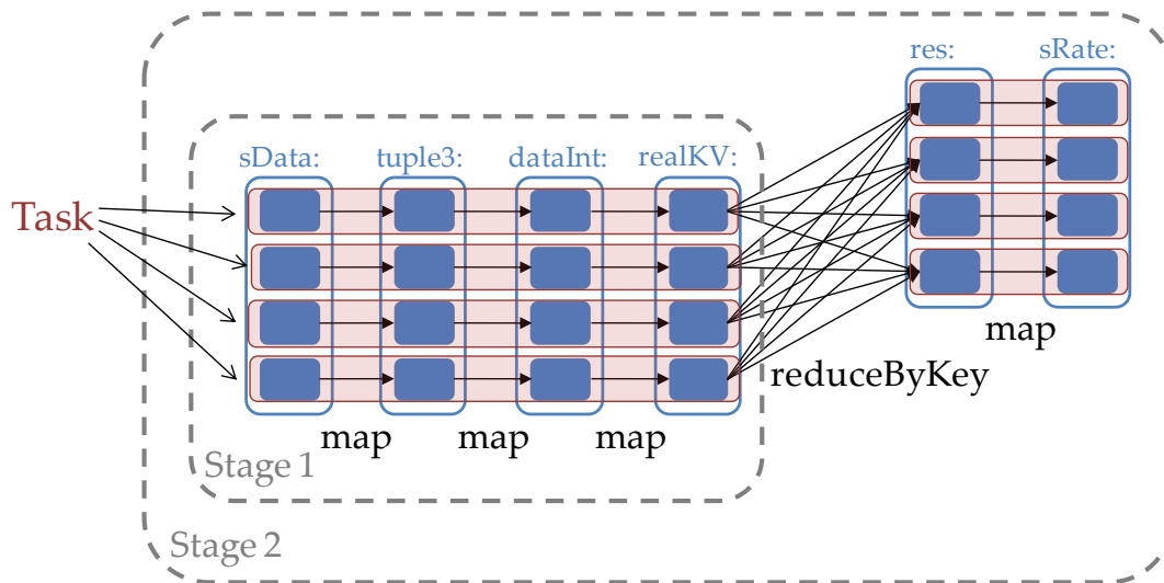
Figura 3: Schema di esecuzione dell'applicazione SongsCount . I box in rosso sono i task, sequenze di istruzioni eseguite da un solo executor.
