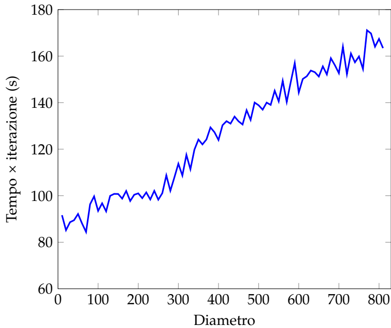
Figura 13: HADI-Spark nel calcolo di road-CA . Tempo impiegato per eseguire un'iterazione del ciclo di HADI al variare del diametro raggiunto.
