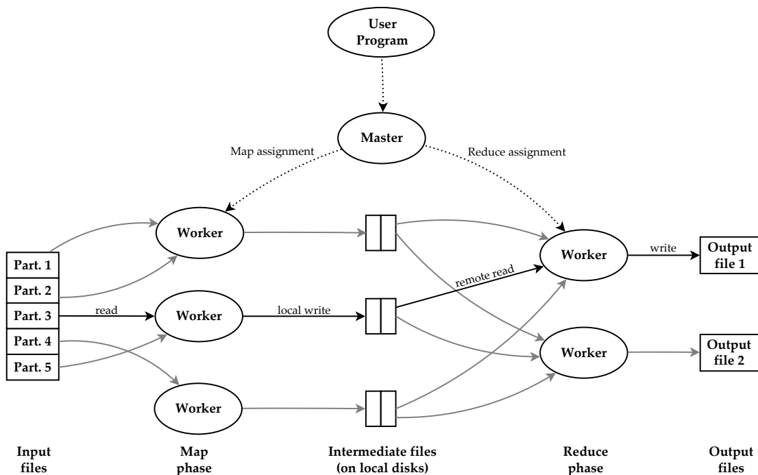
Figura 4: Schema di un'elaborazione MapReduce.
