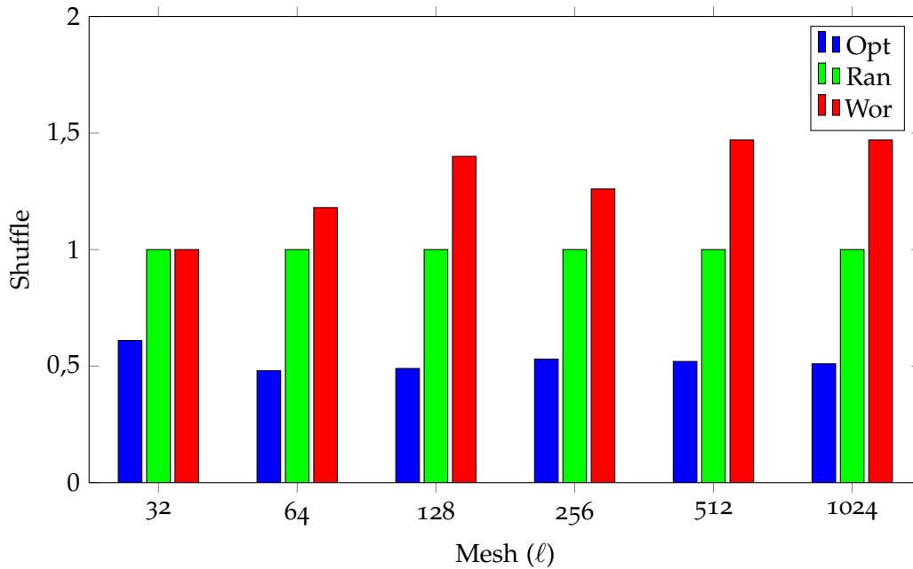
Figura 18: Numero di dati creati per lo shuffle, con diverse mesh e divisi per funzione di ripartizione. Valori normalizzati sulla distribuzione random.
