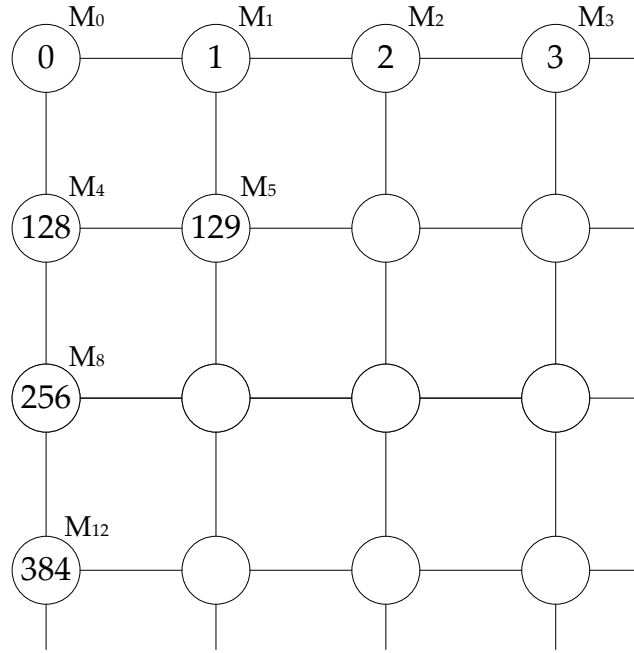
Figura 17: Partizionamento pessimo per una mesh con \ell = 128 .
