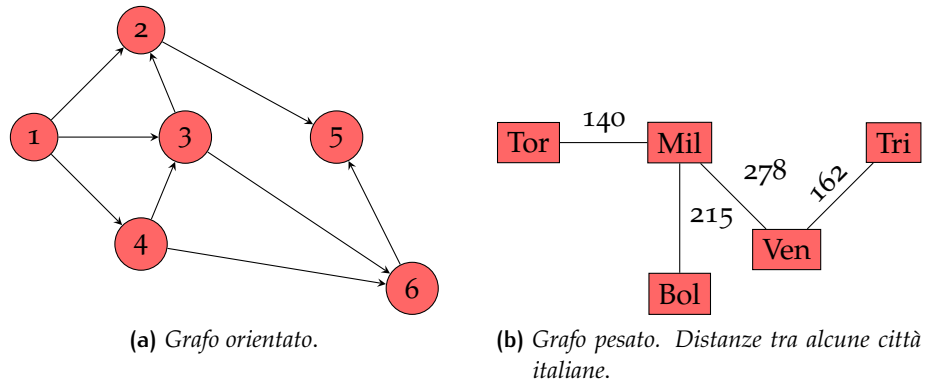
Figura 6: Esempi di grafi.
