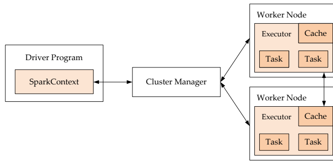
Figura 2: Schema dei componenti di Spark.
