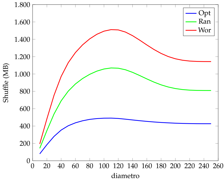
Figura 20: Valori degli shuffle per la mesh 128 \times 128 campionati su tutte le iterazioni di HADI-Spark.
