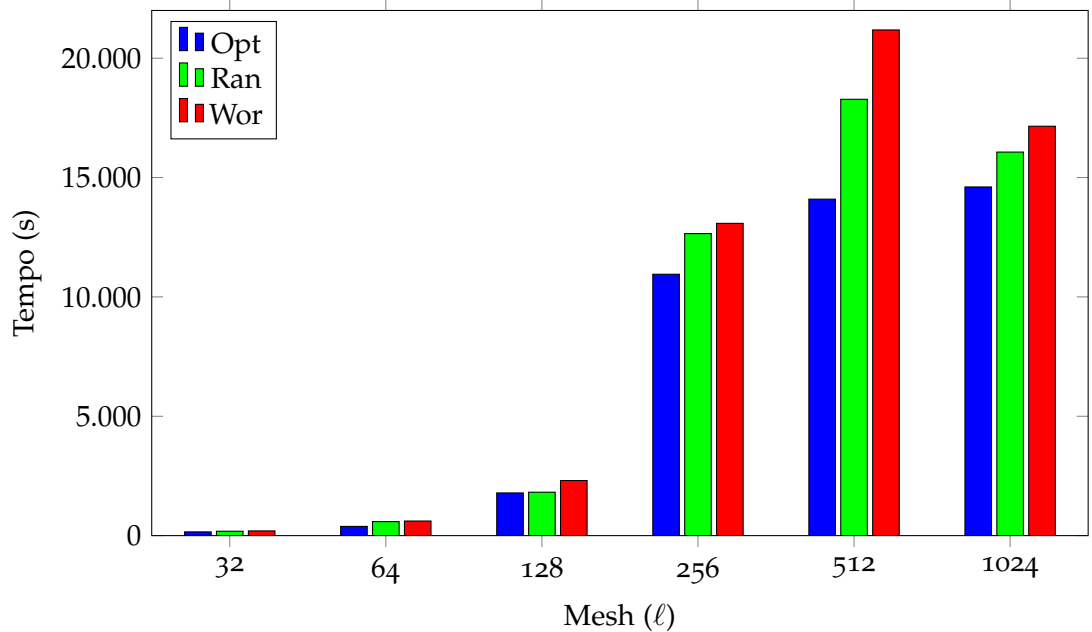
Figura 19: Tempi di esecuzione per l'esperimento in Figura 18. Le misure tra mesh diverse non vanno rapportate tra loro perché sono stati utilizzati numeri di registri diversi.
