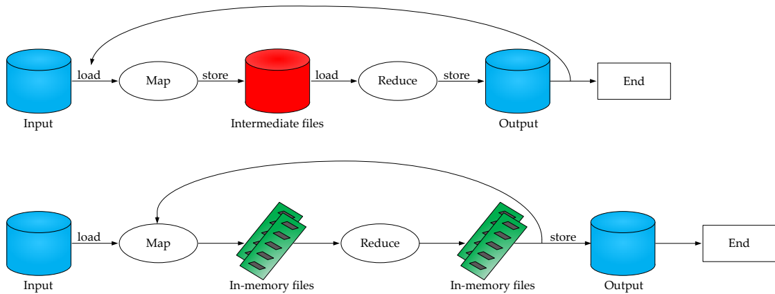
Figura 9: Confronto tra Spark e Hadoop in un ciclo MapReduce.
