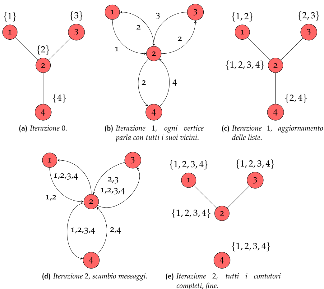
Figura 7: Esempio di calcolo del diametro con HADI. Il diametro è il valore dell'ultima iterazione.
