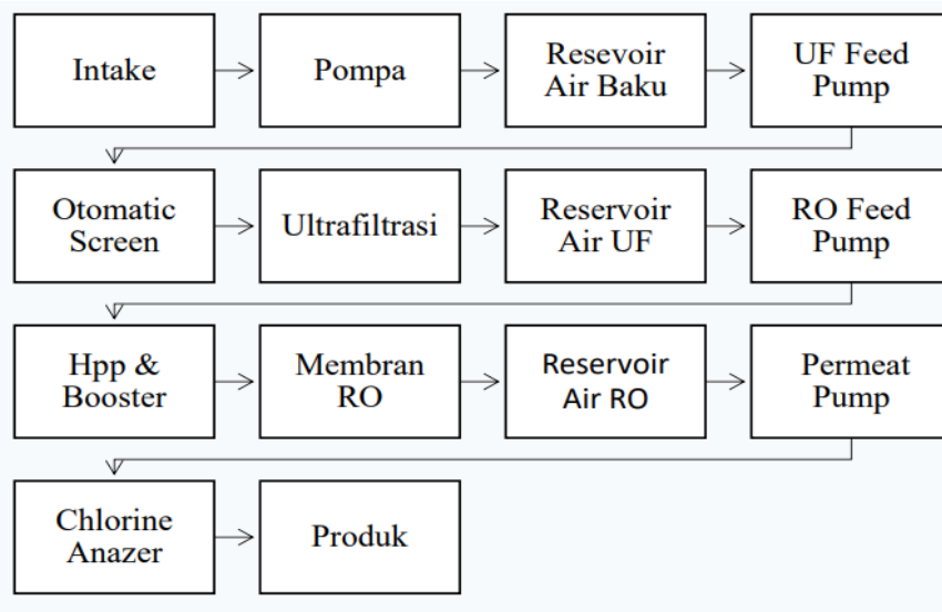
Gambar 2. Proses Desalinasi air laut dengan teknologi Reverse Osmosis (RO) Figure 2. Seawater Desalination Process with Reverse Osmosis technology
